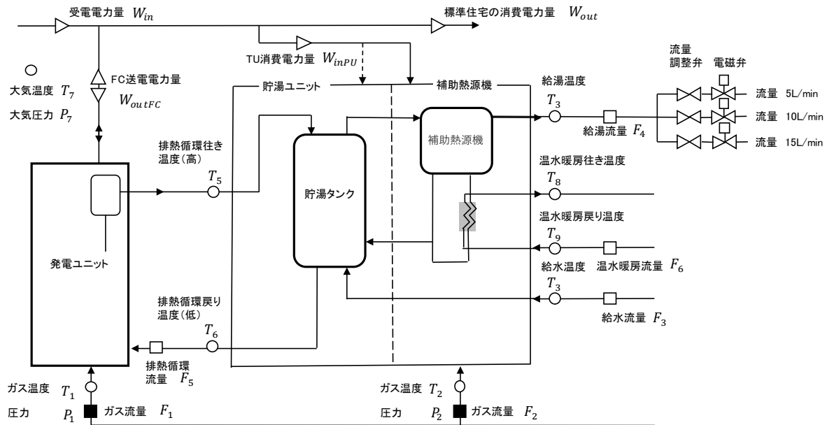
図 5 試験装置及び計測ポイント(例)
